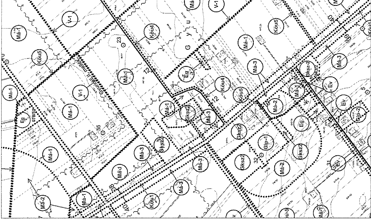
Módosított szabályozási tervrészlet
